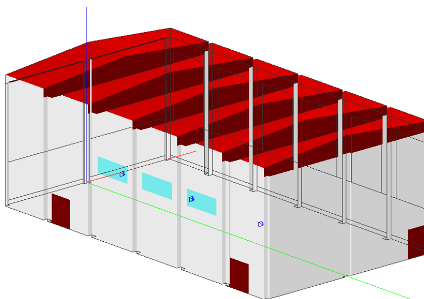
Fig.3 Komputerowy model sali sportowej.
