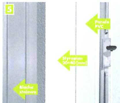
Bramę w wersji z ociepleniem
