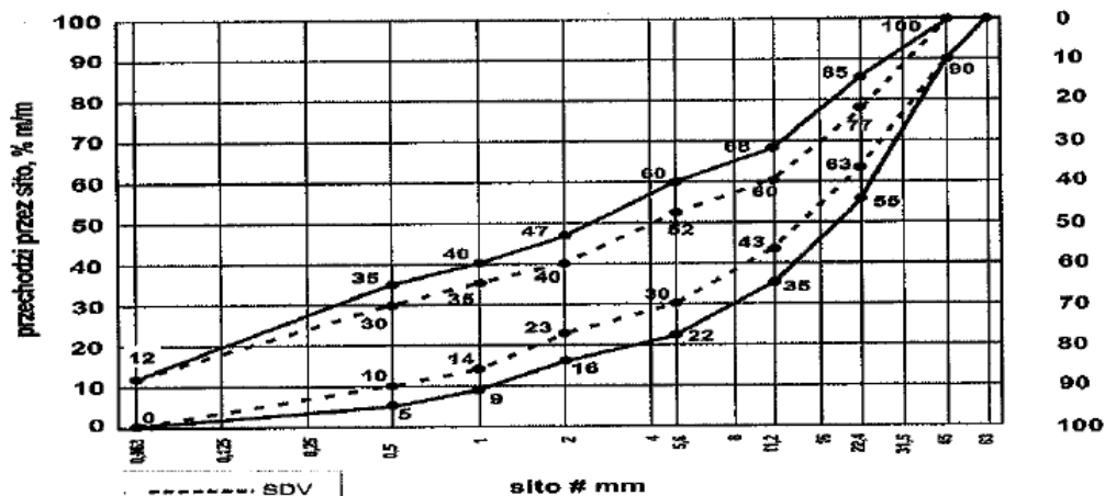
Rys. 2. Mieszanka niezwiązana 0/45 do warstw ulepszonego podłoża
