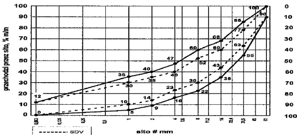
Rys. 3. Mieszanka niezwiązana 0/63 do warstwy ulepszonego podłoża
