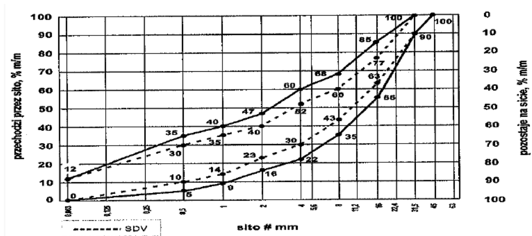
Rys. 1. Mieszanka niezwiązana 0/31,5 do warstw ulepszonego podłoża
