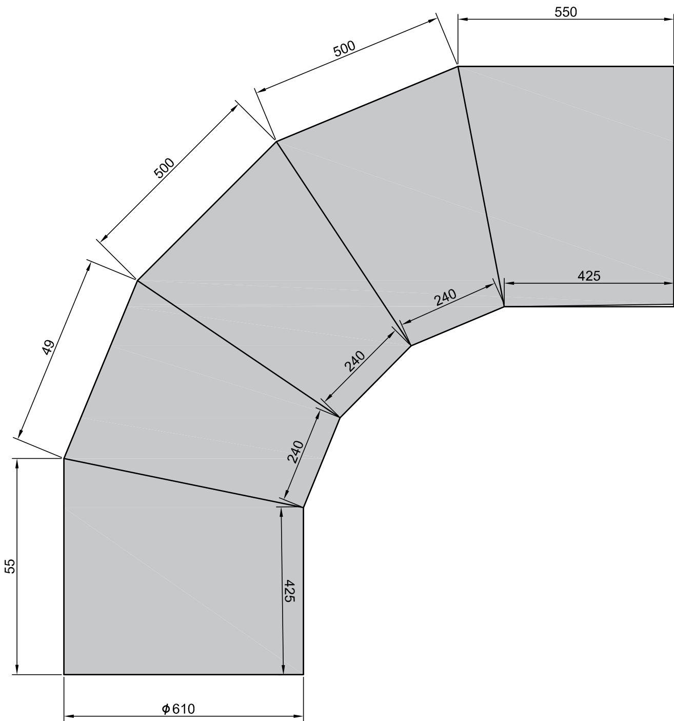
kolano stalowe segmentowe Dn600
