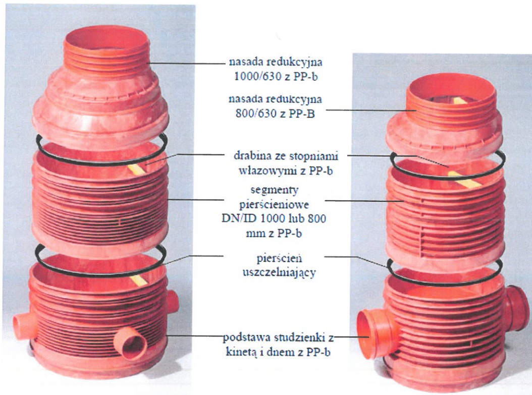
Rys. 3 Studzienka PRO 800
