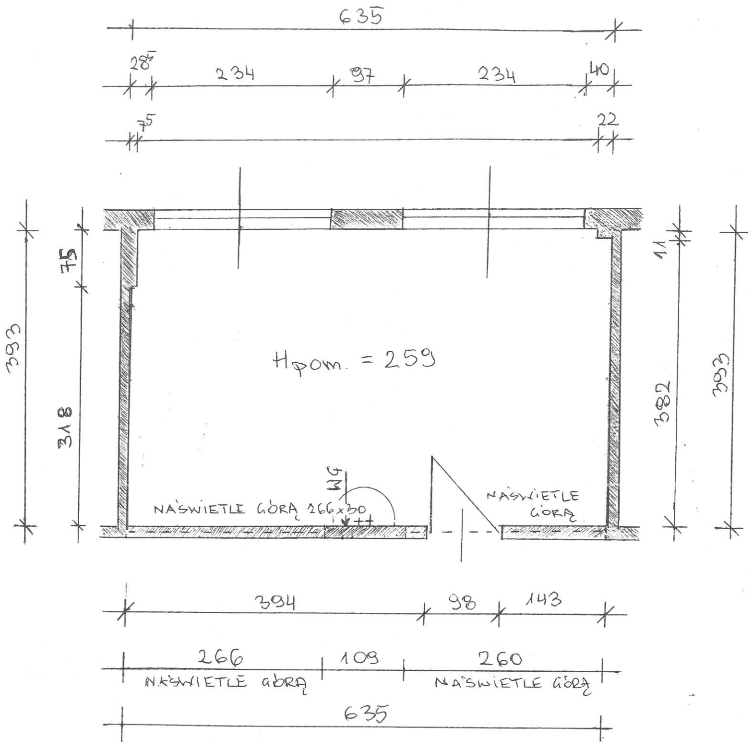
SCHEMAT POMIESZCZENIA SKALA 1:50
