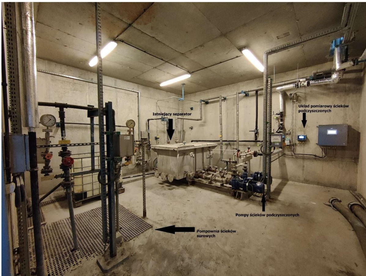
Rysunek. 1. Pomieszczenie pompni.
