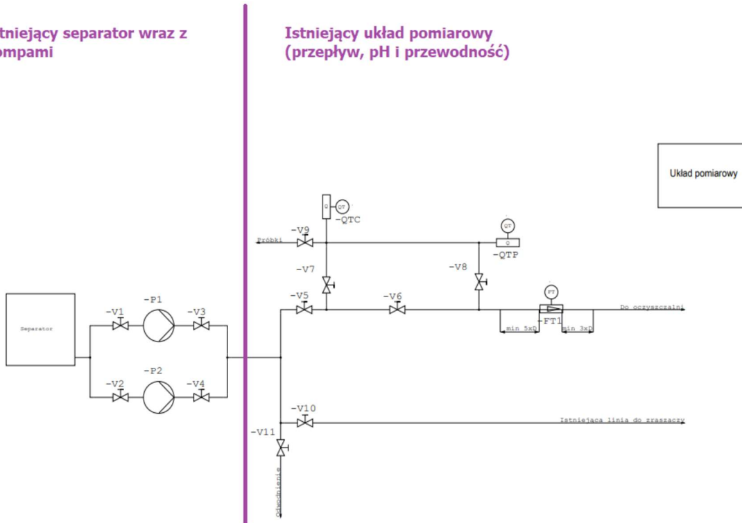
Rysunek. 2. Schemat istniejącego układu pomiarowego zainstalowanego za planowanym urządzeniem podczyszczania ścieków.
