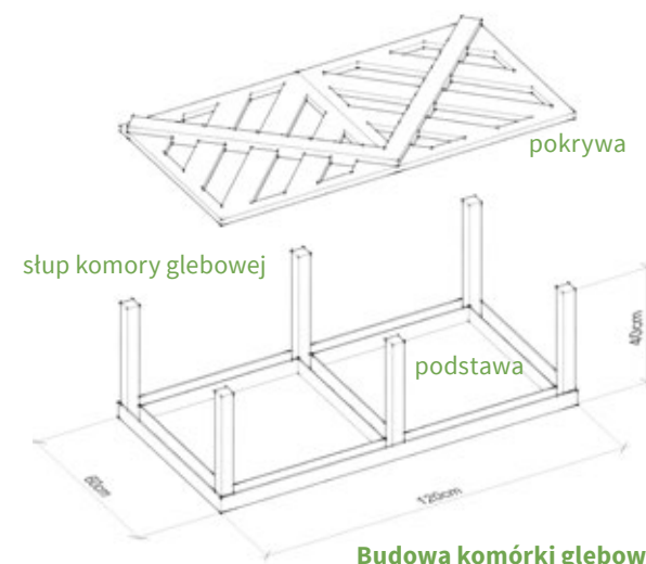
Budowa komórki glebowej
