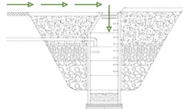
Schemat studni chłonnej z obniżonym osadnikiem
