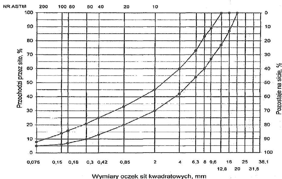
Rys. 13. Krzywe graniczne uziarnienia mieszanki mineralnej BA od 0 do 16 mm do warstwy wyrównawczej i wzmacniającej nawierzchni drogi o obciążeniu ruchem od KR3 do KR6
