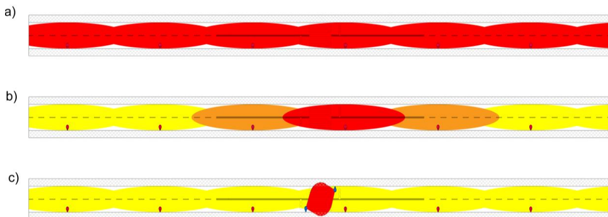
Rys. 1.2 Schemat rozmieszczenia opraw oświetlenia w obszarze przejścia dla pieszych: a) rozwiązanie standardowe b) rozwiązanie standardowe ze strefa przejściową c) rozwiązanie dedykowane Źródło: Opracowanie własne
