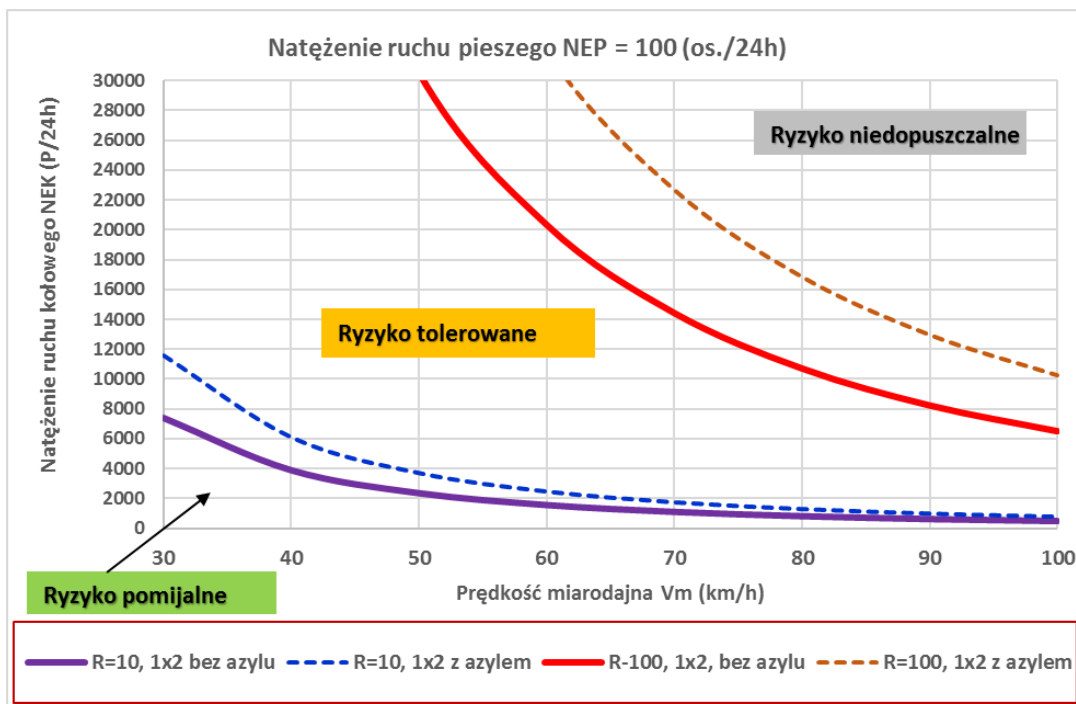
Rys. 9.1 Zakresy akceptowalności ryzyka na przejściu dla pieszych zlokalizowanym na dwupasowej drodze dwukierunkowej, dla natężenia uchu pieszego NEP = 100 os. 24 h Źródło: Opracowanie własne
