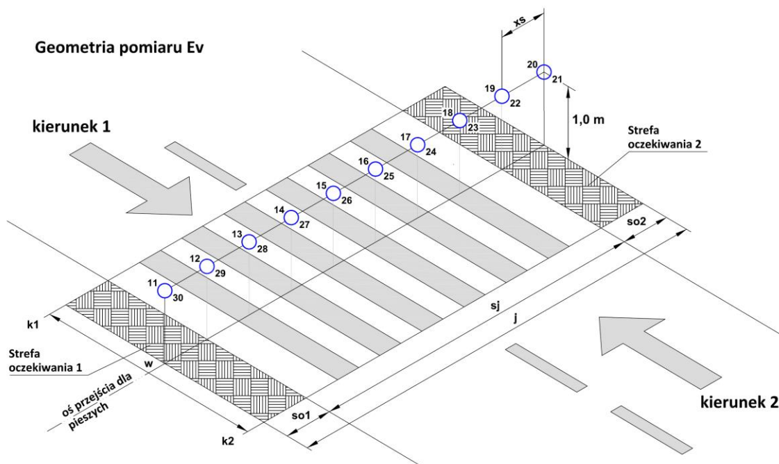
Rys. 6.1 Przykładowe rozmieszczenie punktów pomiarowych natężenia oświetlenia w płaszczyźnie pionowej ( E_v ) na przejściu dla pieszych stosowana w procedurze kontrolnej Źródło: Opracowanie własne
