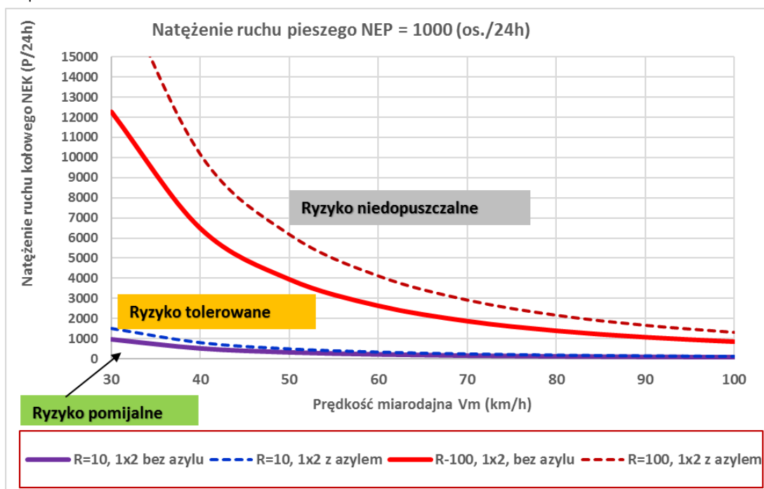
Rys. 9.2 Zakresy akceptowalności ryzyka na przejściu dla pieszych zlokalizowanym na dwupasowej drodze dwukierunkowej, dla natężenia uchu pieszego NEP = 1000 os. 24 h Źródło: Opracowanie własne
