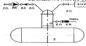
SCHEMAT PODŁĄCZENIA ODGAZOWYWACZY TERMICZNYCH TYP II DO INSTALACJI
