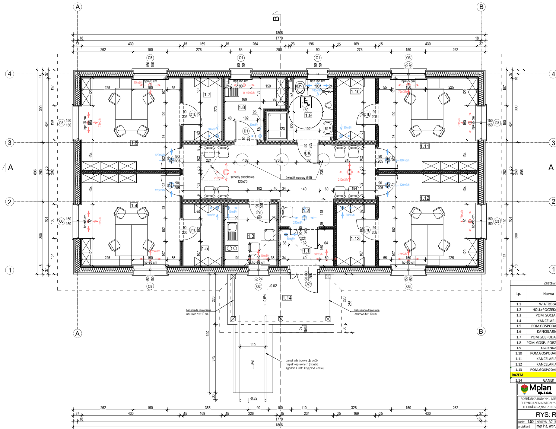
Rzut parteru 1:50
