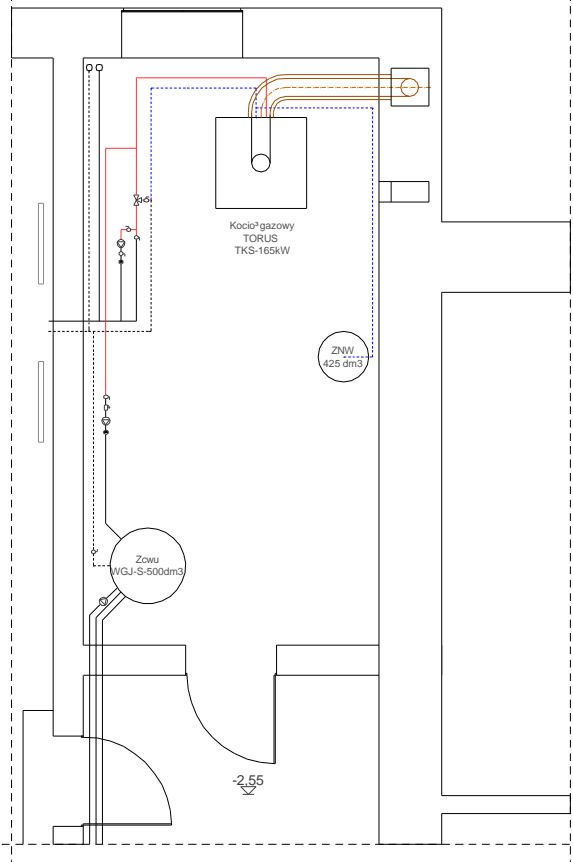
RZUT KOTŁOWNI skala - 1:25
