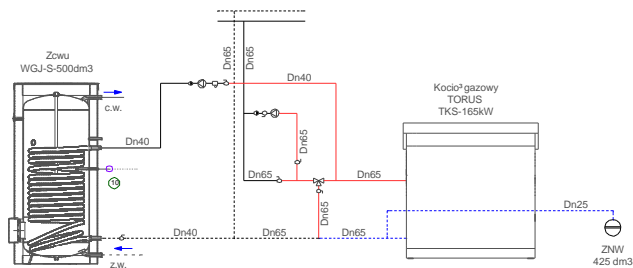
SCHEMAT TECHNOLOGICZNY KOTŁOWNI
