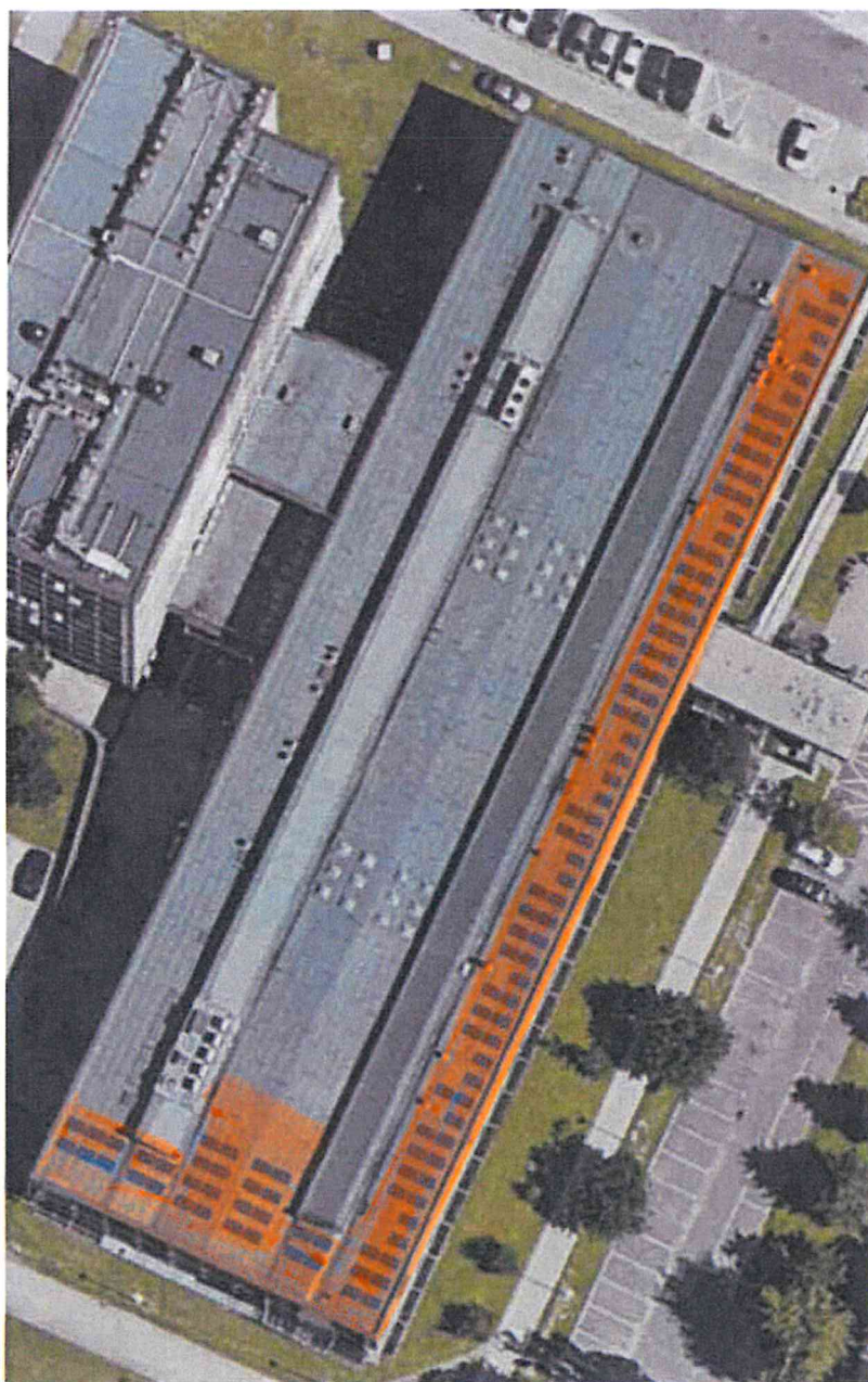
Rys. 2.4.1 Rozmieszczenie modułów PV na dachu budynku.
