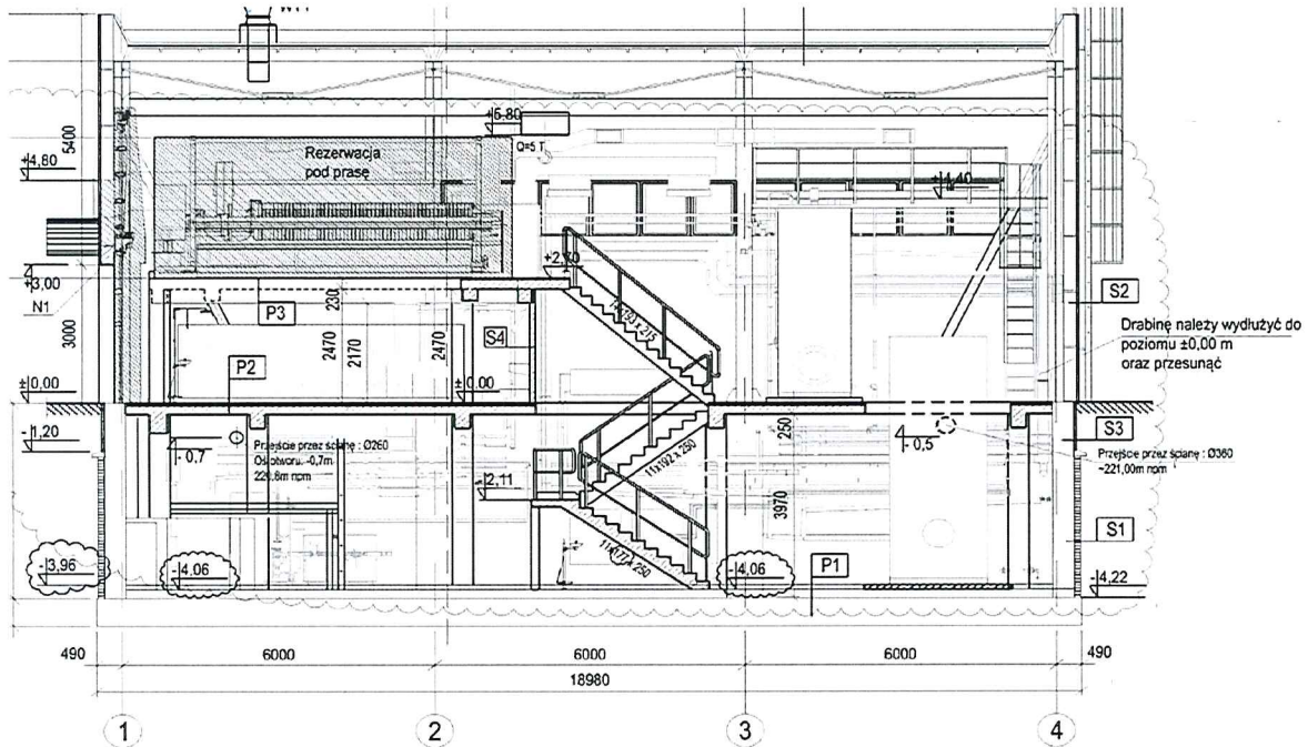
Rys. 2 Przekrój budynku Oczyszczalni Ścieków z wyszczególnionym miejscem pod zabudowę prasy
