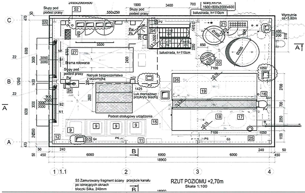
Rys. 1 Rzut poziomu +2,70m Oczyszczalni Ścieków Przemysłowych z miejscem do zabudowy prasy
