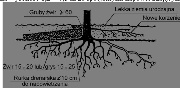
Rys. 5. Studzienka zabezpieczająca pień drzewa przy podwyższeniu terenu powyżej 0,5 m
