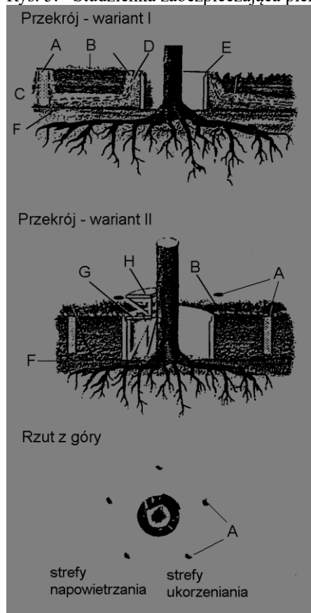
Rys. 5. Studzienka zabezpieczająca pień drzewa przy podwyższeniu terenu powyżej 0,5 m
