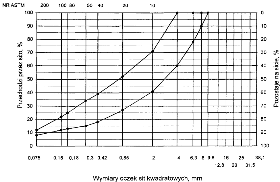
warstwy ścieralnej nawierzchni drogi o obciążeniu ruchem KR1 lub KR2 Rys. 3. Krzywe graniczne uziarnienia mieszanki mineralnej BA od 0 do 8mm, od 0 do 6,3 mm do warstwy ścieralnej nawierzchni drogi o obciążeniu ruchem nawierzchni drogi o obciążeniu ruchem KR1 lub KR2
