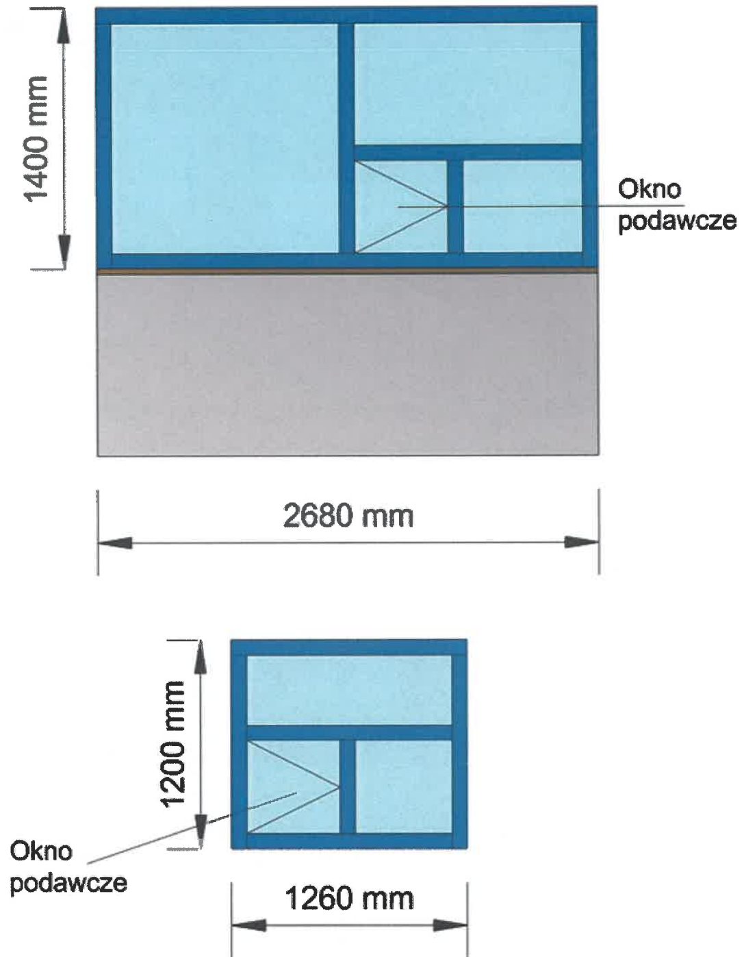
Rysunek poglądowy zabudowy dyżurki w KPP w Legionowie
