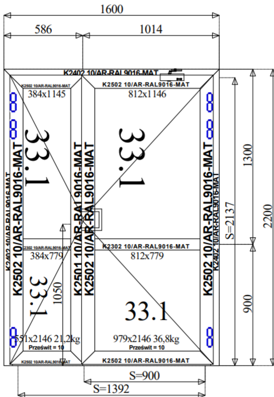
Poz. 1 ACS 50 - drzwi otwierane na zewnątrz (B=1 600, H=2 200)
