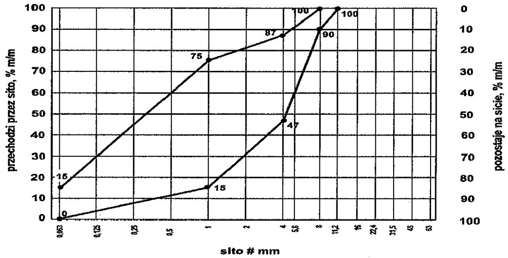
Rys. 1. Krzywe graniczne uziarnienia mieszanki kruszyw 0/8 mm do górnej warstwy podłoża ulepszanego
