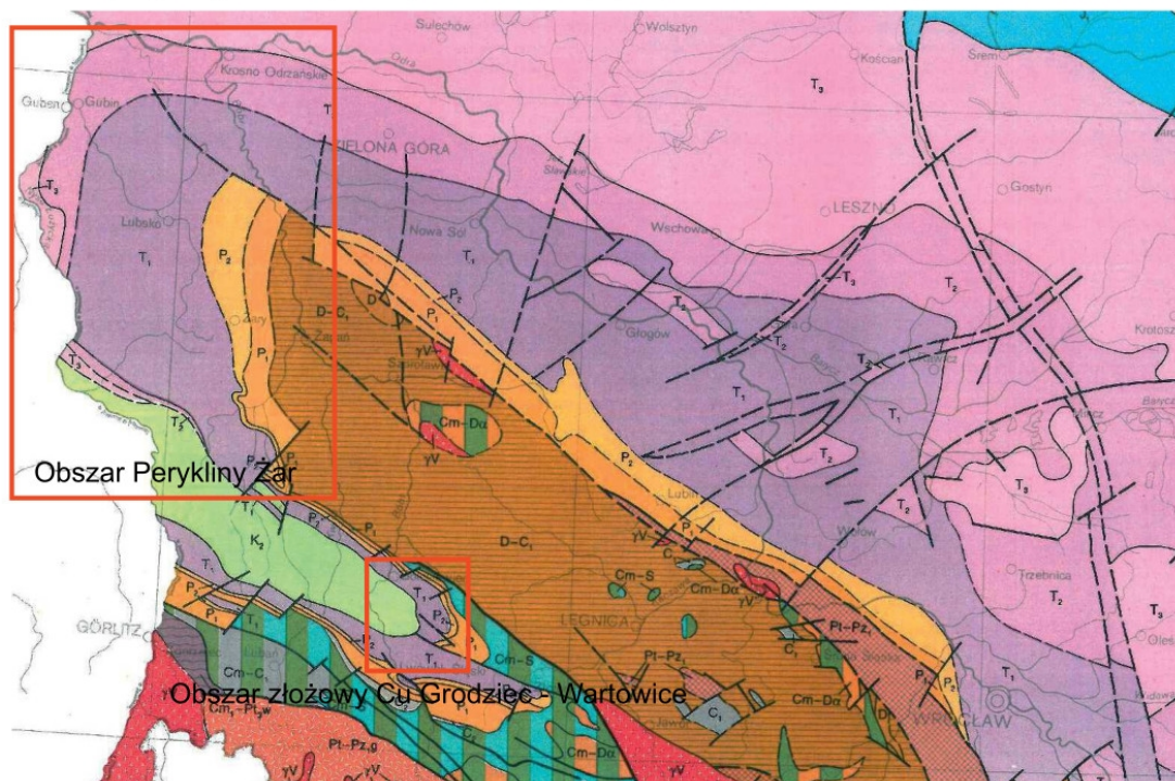
Ryc. 1 Mapa geologiczna ścienia na poziomie 500 m p.p.m. wraz z zaznaczonymi obszarami, które mają być przedmiotem opracowania.
