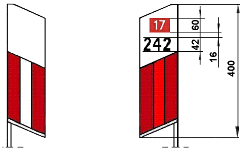
Rys. 2. Słupek prowadzący U-1b z naniesionym znakiem kilometrowym i hektometrym, przeznaczony do umieszczenia na barierze ochronnej, w hektometrze zerowym
