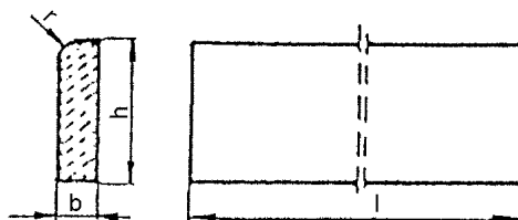
Rysunek 1. Kształt betonowego Tabelica 1. Wymiary obrzeży
