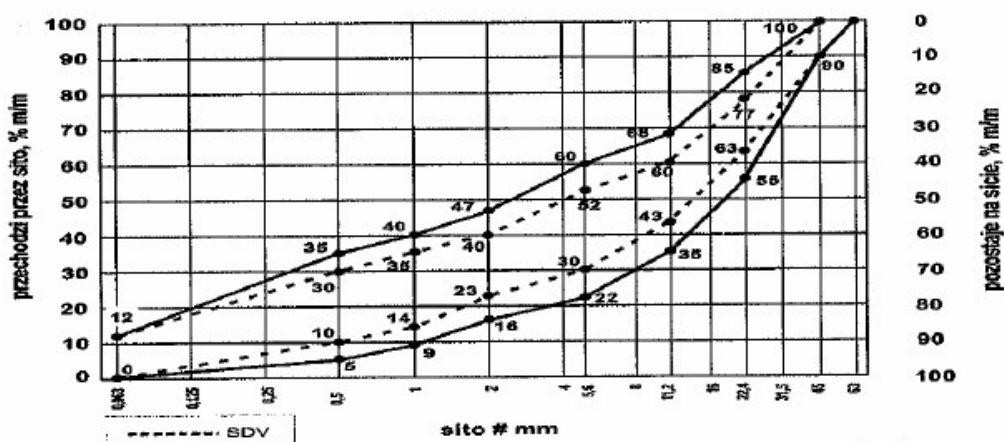
Rys. 9. Krzywe graniczne uziarnienia mieszanki niezwiązanej 0/45 mm do podbudowy pomocniczej
