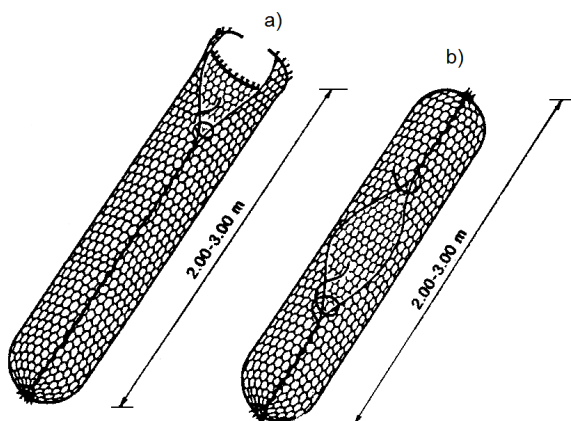
Rys. 10. Worki gabionowe
