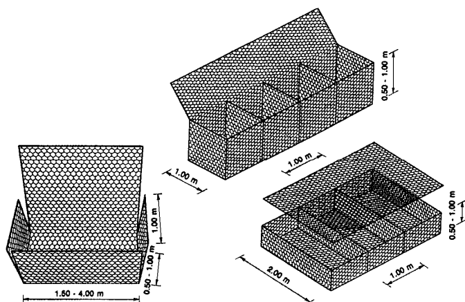
b) Przy rozkładaniu koszy, ściany łączą się szpilką układaną w zsunięte przenikające się spirale dwóch ścian lub spinaczem zaciśniętym zszywarką (można też użyć drutu wiązkowego)
