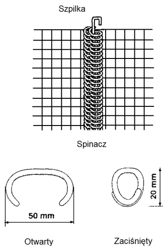
b) Przy rozkładaniu koszy, ściany łączą się szpilką układaną w zsunięte przenikające się spirale dwóch ścian lub spinaczem zaciśniętym zszywarką (można też użyć drutu wiązkowego)
