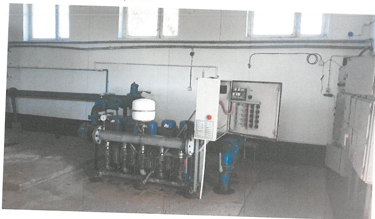
Zestaw hydroforowy wody na sieć
