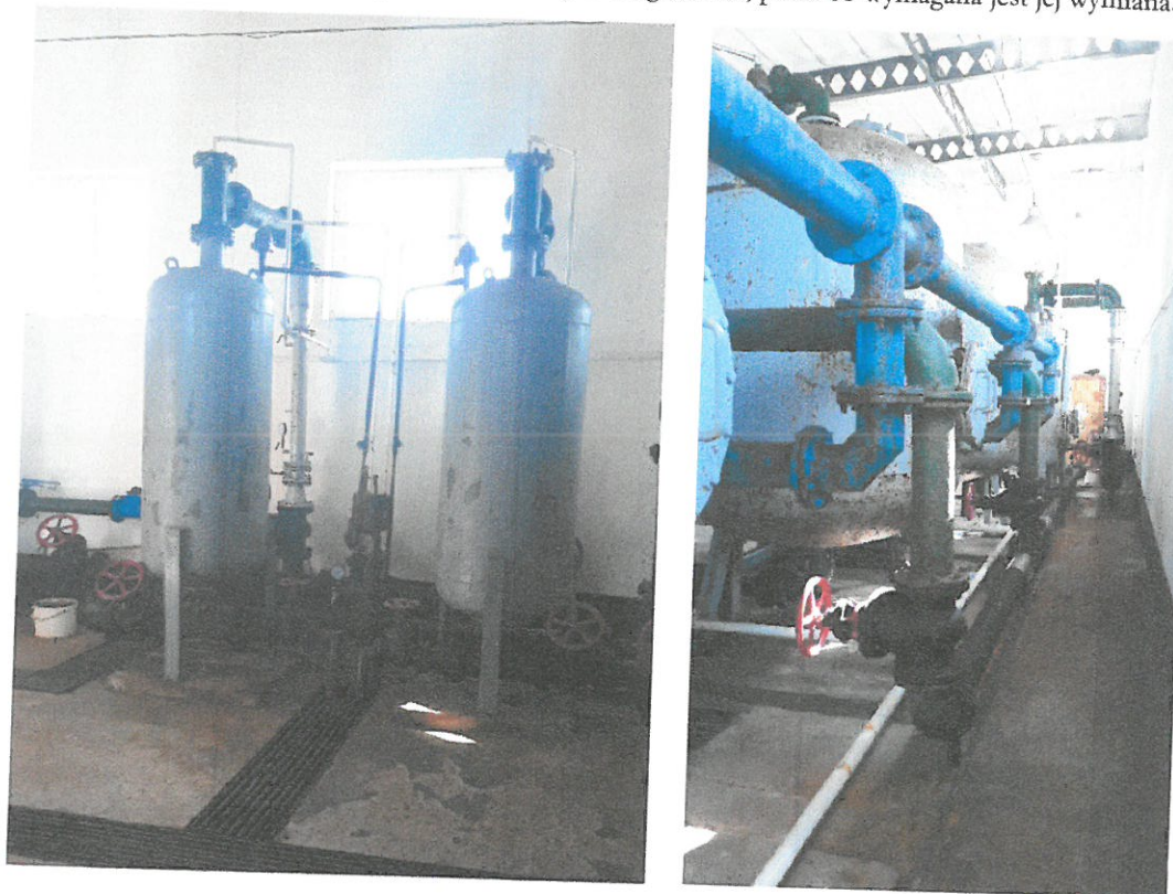
Aeratory , rurociągi technologiczne
