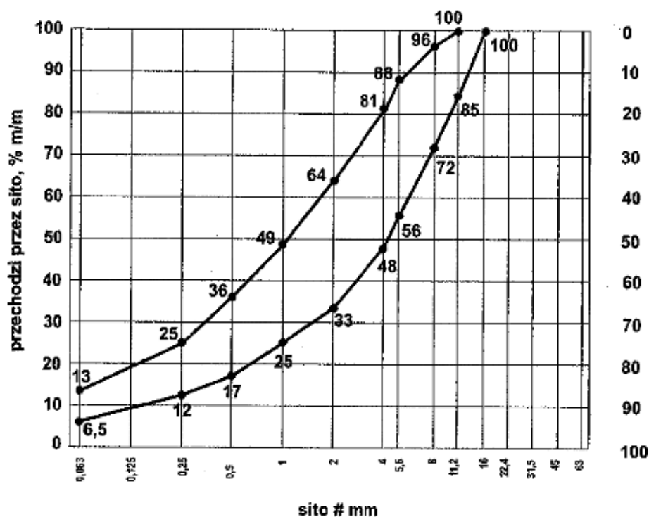
Rys. 4. Krzywe graniczne uziarnienia mieszanki mineralnej 0/11,2 mm
