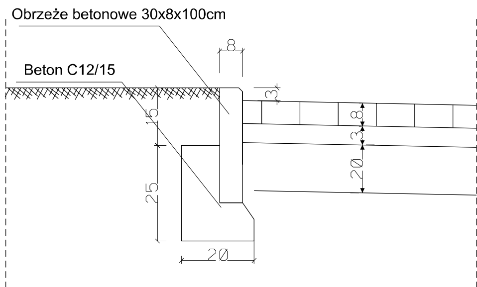
Szczegół konstrukcyjny 1
