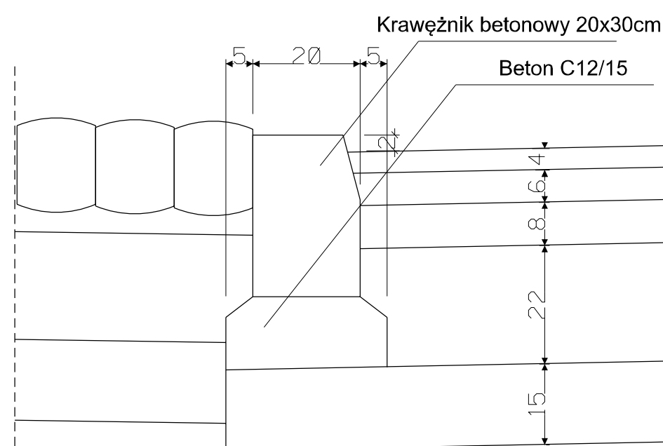
Szczegół konstrukcyjny 3
