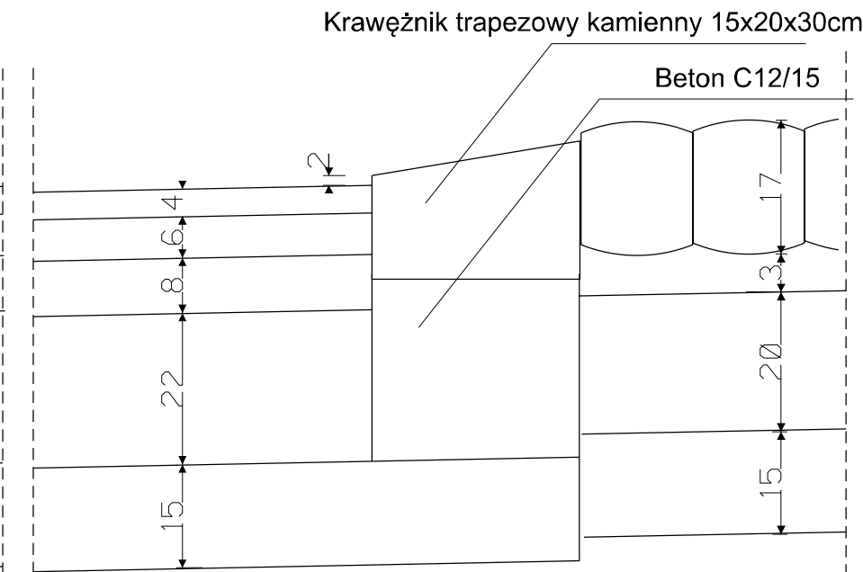
Szczegół konstrukcyjny 4
