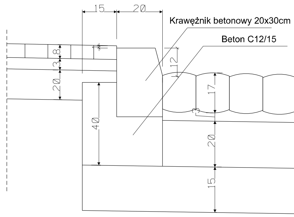
Szczegół konstrukcyjny 2
