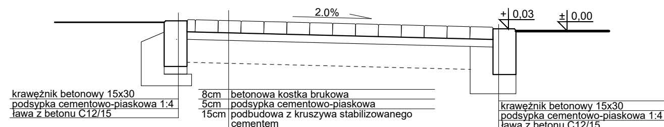
PROFIL POPRZECZNY ZJAZDU
