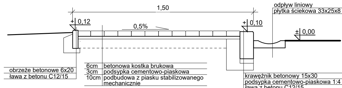
PROFIL POPRZECZNY CHODNIKA B-B
