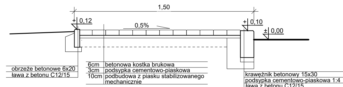
PROFIL POPRZECZNY CHODNIKA A-A
