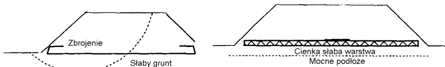
a - zbrojenie podstawy nasypu b - materac w podstawie nasypu Rys. 2.2. Przykłady zbrojenia nasypów geosyntetykami
