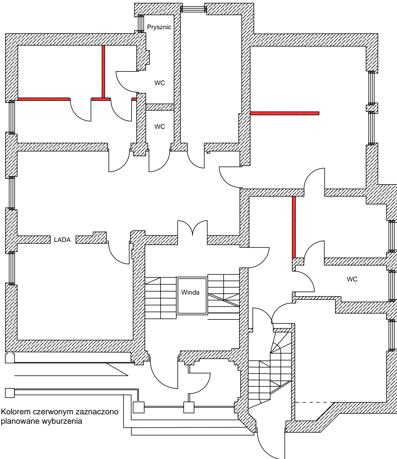
Rzut Parteru
