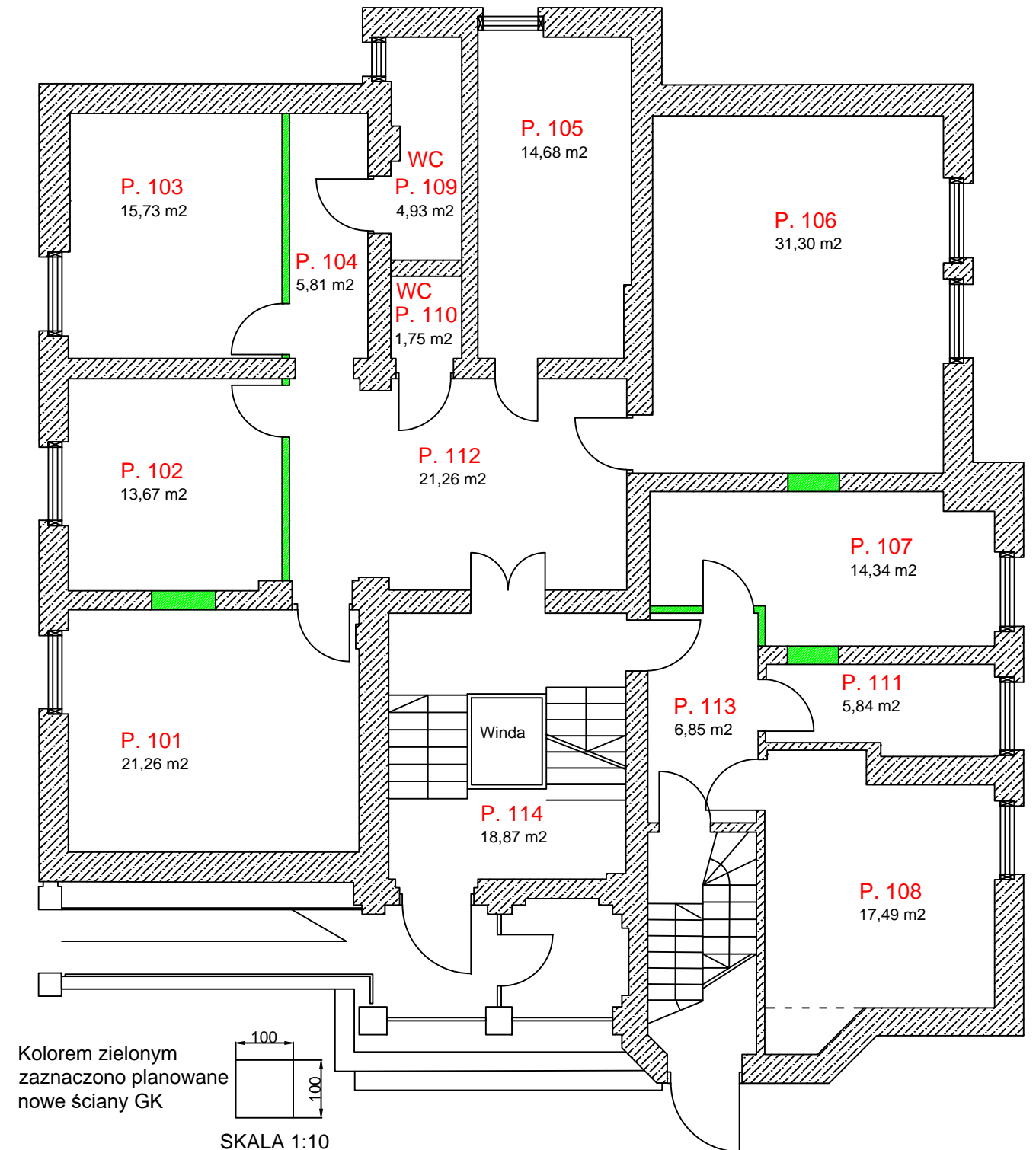
Rzut Parteru
