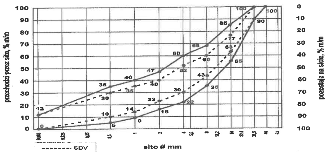
Rys. 1. Mieszanka niezwiązana 0/31,5 do warstw podbudowy
