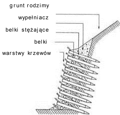
Przekrój poprzeczny kaszycy (Begemann i Schiechtel 1999)
