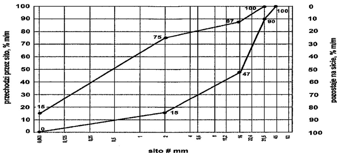
Rys. 1. Mieszanka niezwiązana 0/31,5 do warstwy ulepszonego podłoża
