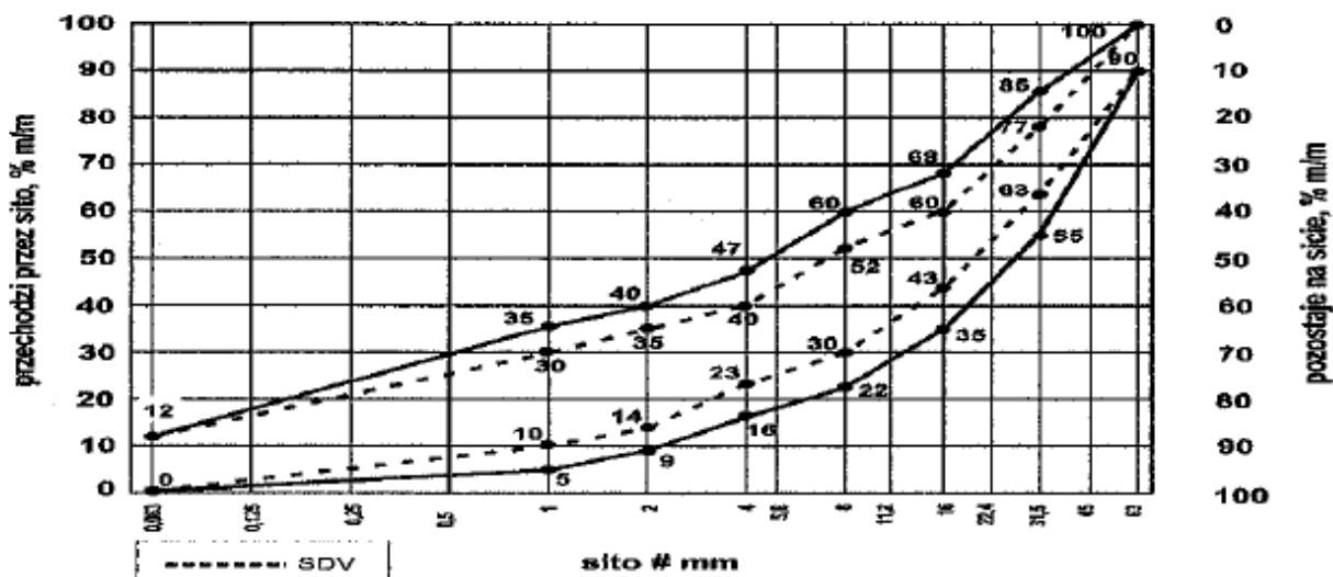
Rys. 3. Mieszanka niezwiązana 0/63 do warstwy podbudowy pomocniczej
