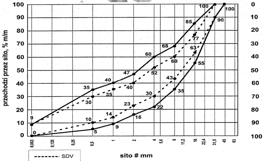
Rys. 2. Mieszanka niezwiązana 0/31,5 do warstwy podbudowy zasadniczej
