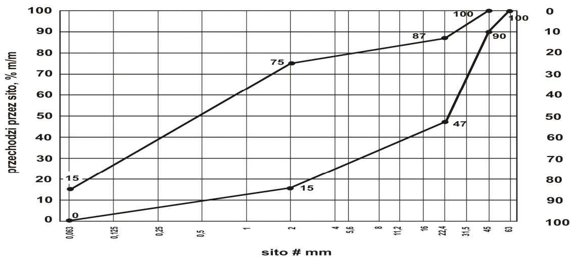
Rys. 6. Uziarnienie mieszanki niezwiązanej 0/45 dla nawierzchni
