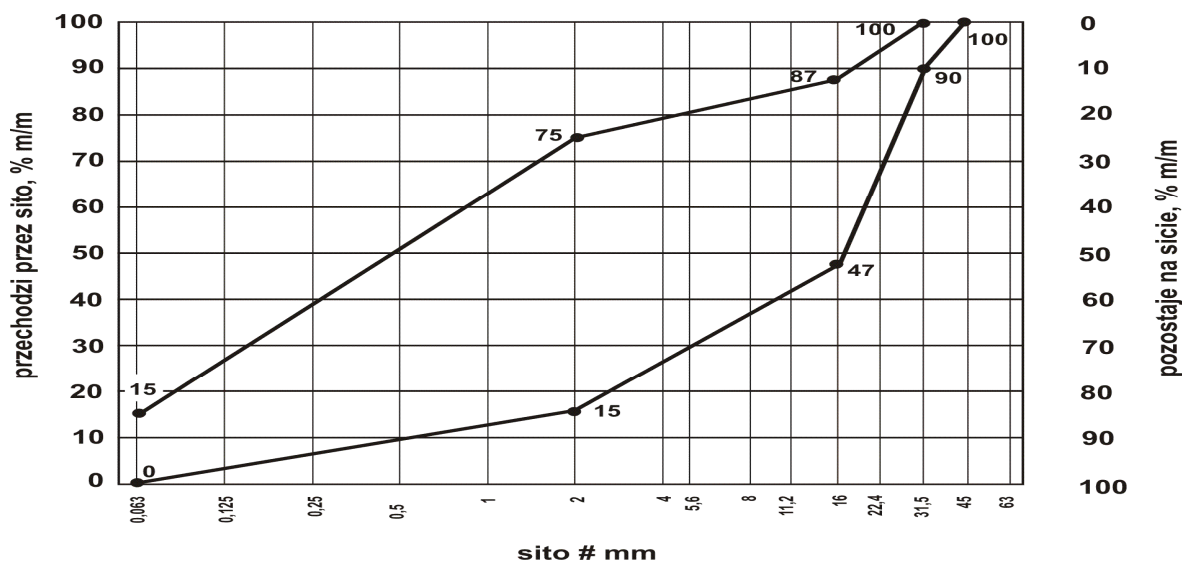
Rys. 5. Uziarnienie mieszanki niezwiązanej 0/31,5 dla nawierzchni
