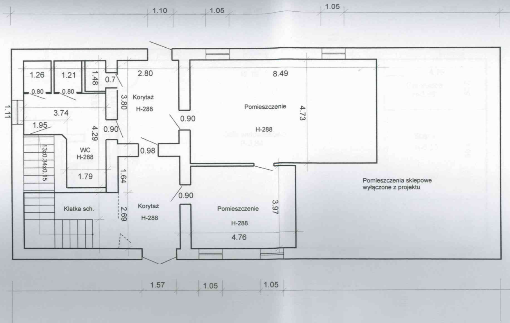
Inwentaryzacja- rzut parteru Dom Ludowy- Zielęcice
