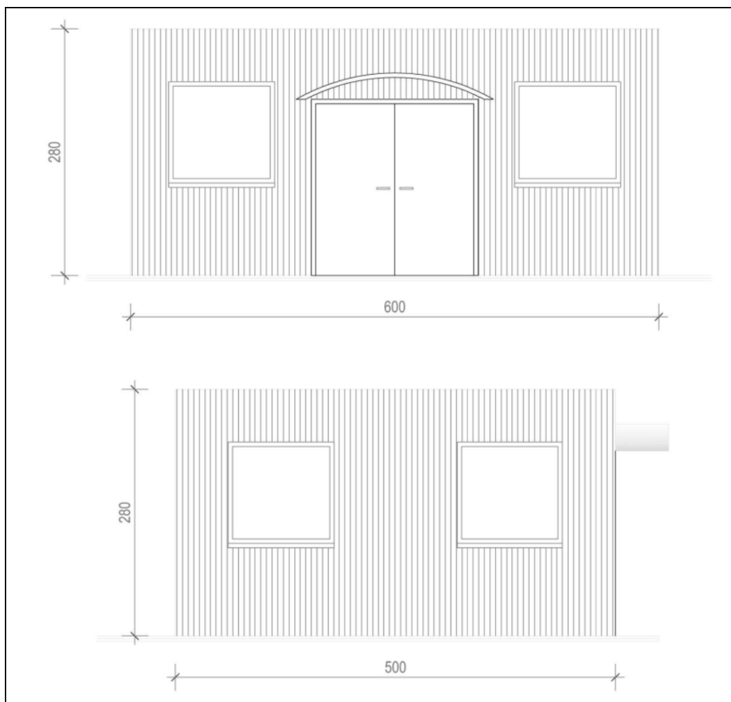
Ryc. 11. Elewacja przednia i boczna magazynu
