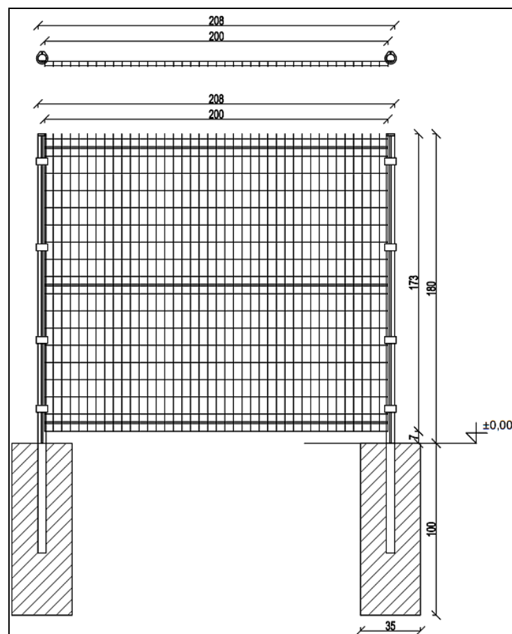
Ryc. 15. Schemat panelu ogrodzeniowego z fundamentem
