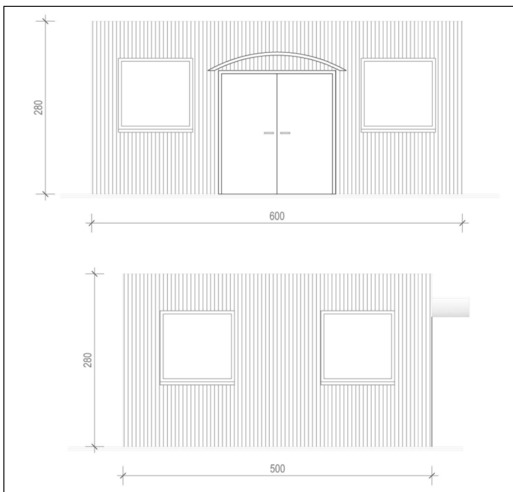
Ryc. 9. Elewacja przednia i boczna magazynu
