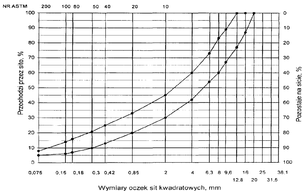
Wymiary oczek sit kwadratowych, mm Rys. 12. Krzywe graniczne uziarnienia mieszanki mineralnej BA od 0 do 20 mm do warstwy wiążącej, wyrównawczej i wzmacniającej nawierzchni drogi o obciążeniu ruchem od KR3 do KR6
