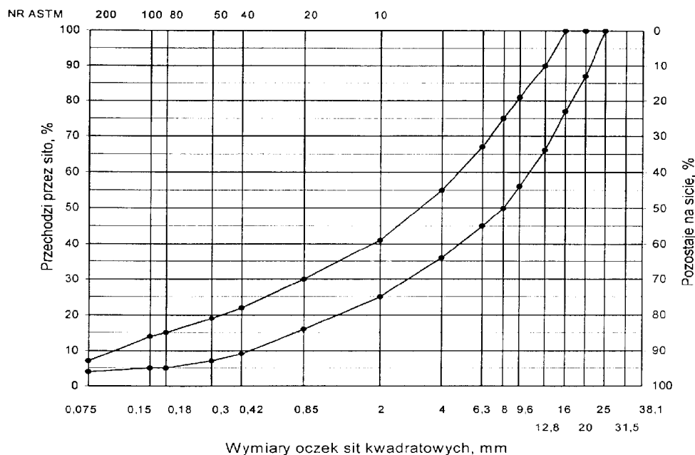
Wymiary oczek sit kwadratowych, mm Rys. 12. Krzywe graniczne uziarnienia mieszanki mineralnej BA od 0 do 20 mm do warstwy wiążącej, wyrównawczej i wzmacniającej nawierzchni drogi o obciążeniu ruchem od KR3 do KR6
