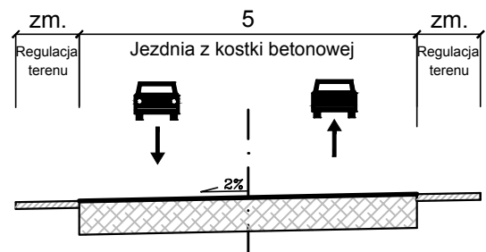
PRZEKRÓJ C - C
