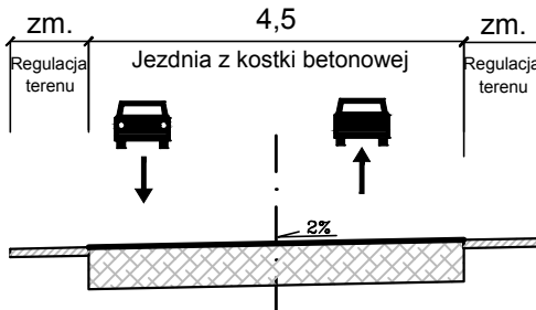
PRZEKRÓJ D - D
