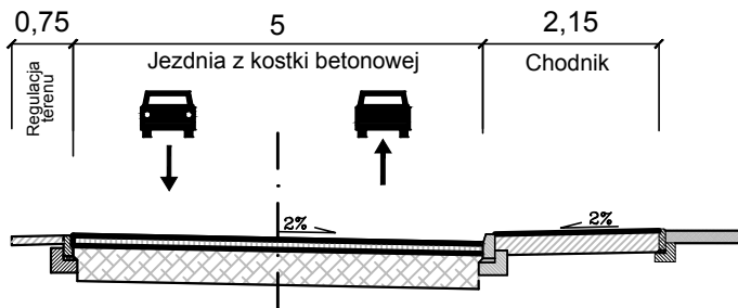
PRZEKRÓJ B - B
