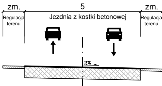
PRZEKRÓJ B - B
