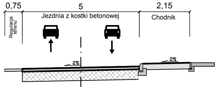
PRZEKRÓJ E - E
