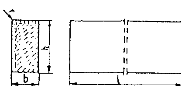
Rys. 1. Wymiarowanie krawężników
