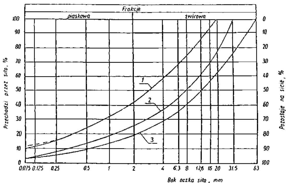
Rysunek 1. Pole dobrego uziamienia kruszyw przeznaczonych na podbudowy wykonywane metodą stabilizacji mechanicznej
