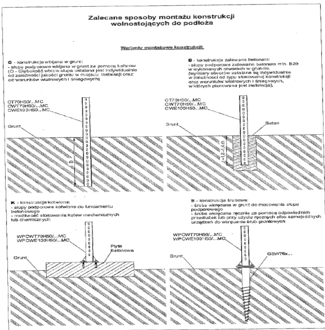
Rysunek 3. Sposoby montażu konstrukcji do podłoża.
