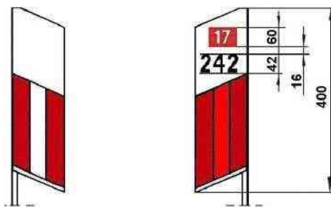
Rys. nr 1 Słupek prowadzący U-lb z naniesionym znakiem kilometrowym i hektometrowym oraz numerem drogi przeznaczony do umieszczenia na barierze ochronnej, w hektometrze zerowym
