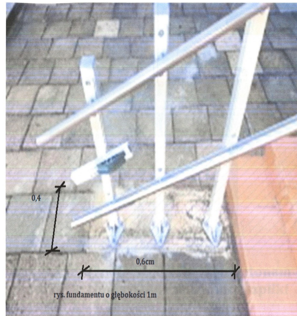
Rys 1 . Zdjęcie poglądowe z przygotowania fundamentu o wymiarach 0,4x0,6x1,0 schowanego pod płytą chodnikową.
