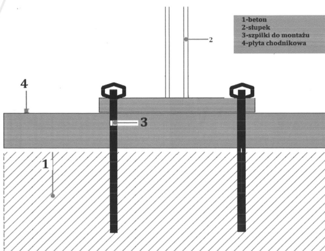
Rys. Szczegół połączenia słupka z betonem przez płytę chodnikową za pomocą szpilki
