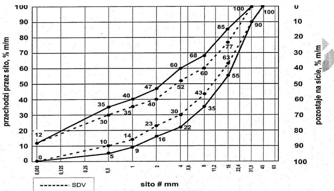
Rys. 1. Mieszanka niezwiązana 0/31,5 do warstwy podbudowy zasadniczej
