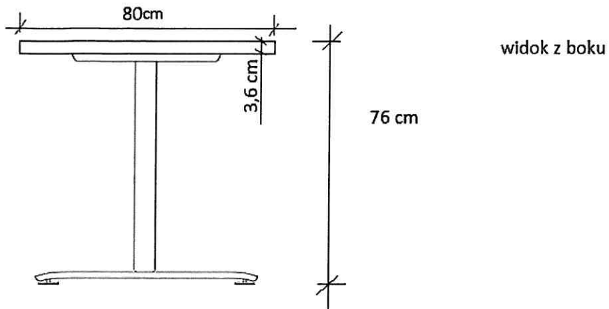
Rys. 12 stół 80 x 180 cm na stelażu metalowym
