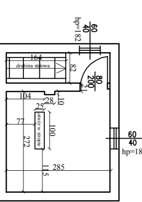
Rzut nadszybia windy
