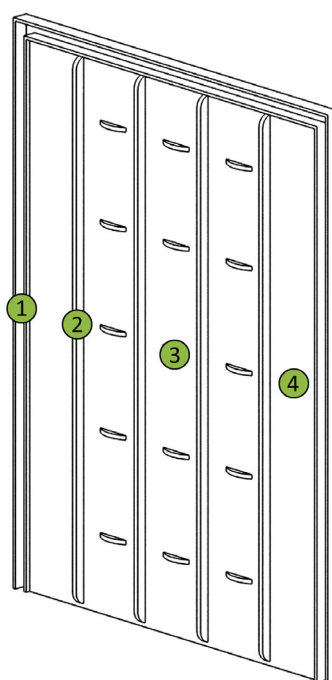
Ryc.14. Schemat pojedynczego panelu bariery mechanicznej (opracowanie własne na podstawie materiałów firmy DeepRoot)
