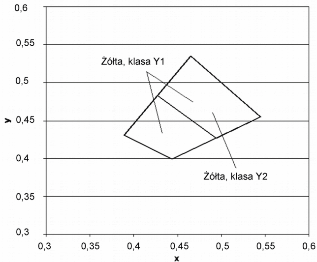
Rys.2. Współrzędne chromatycy x,y dla barwy żółtej oznakowania
