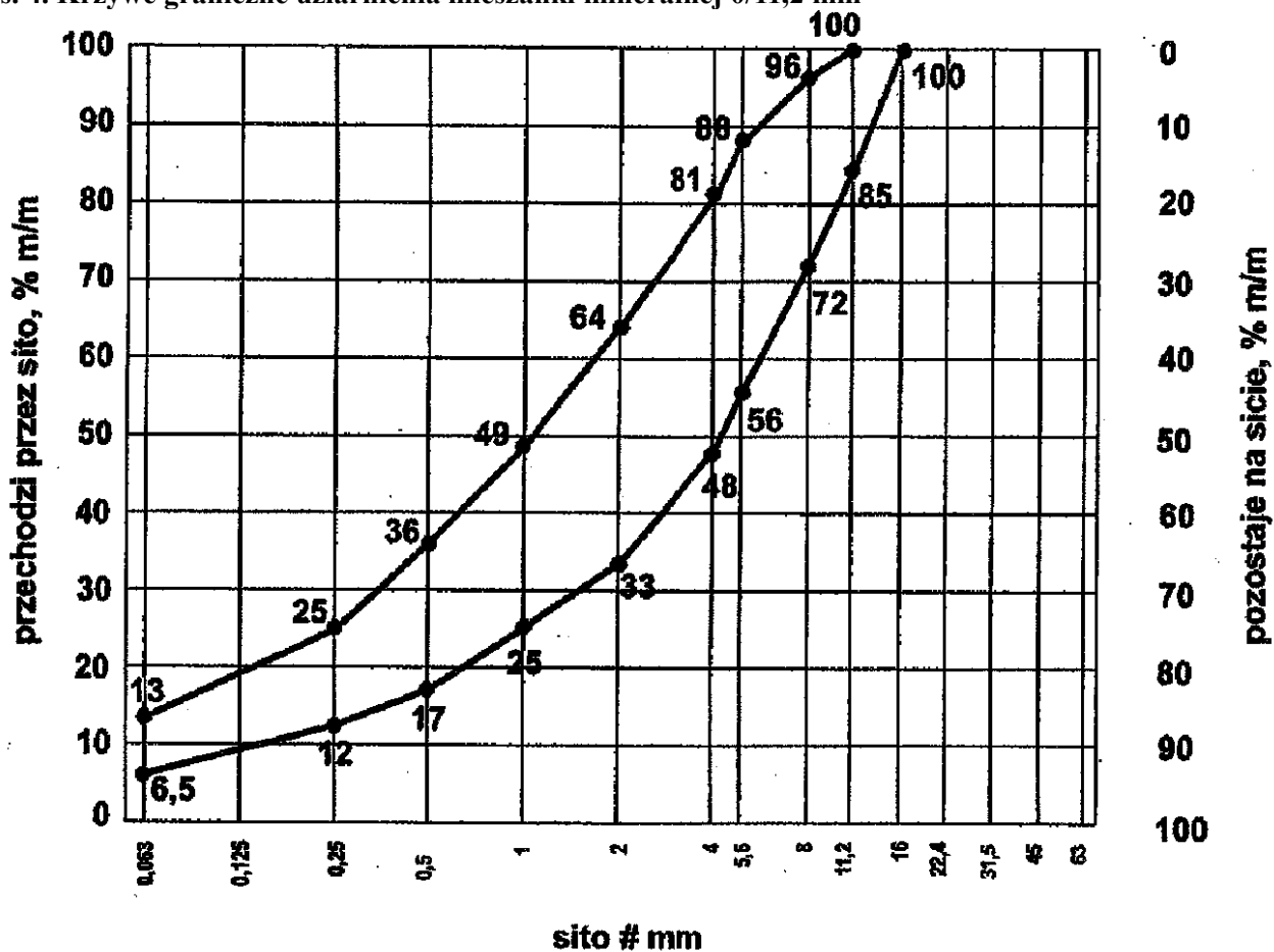
Rys. 4. Krzywe graniczne uziarnienia mieszanki mineralnej 0/11,2 mm
