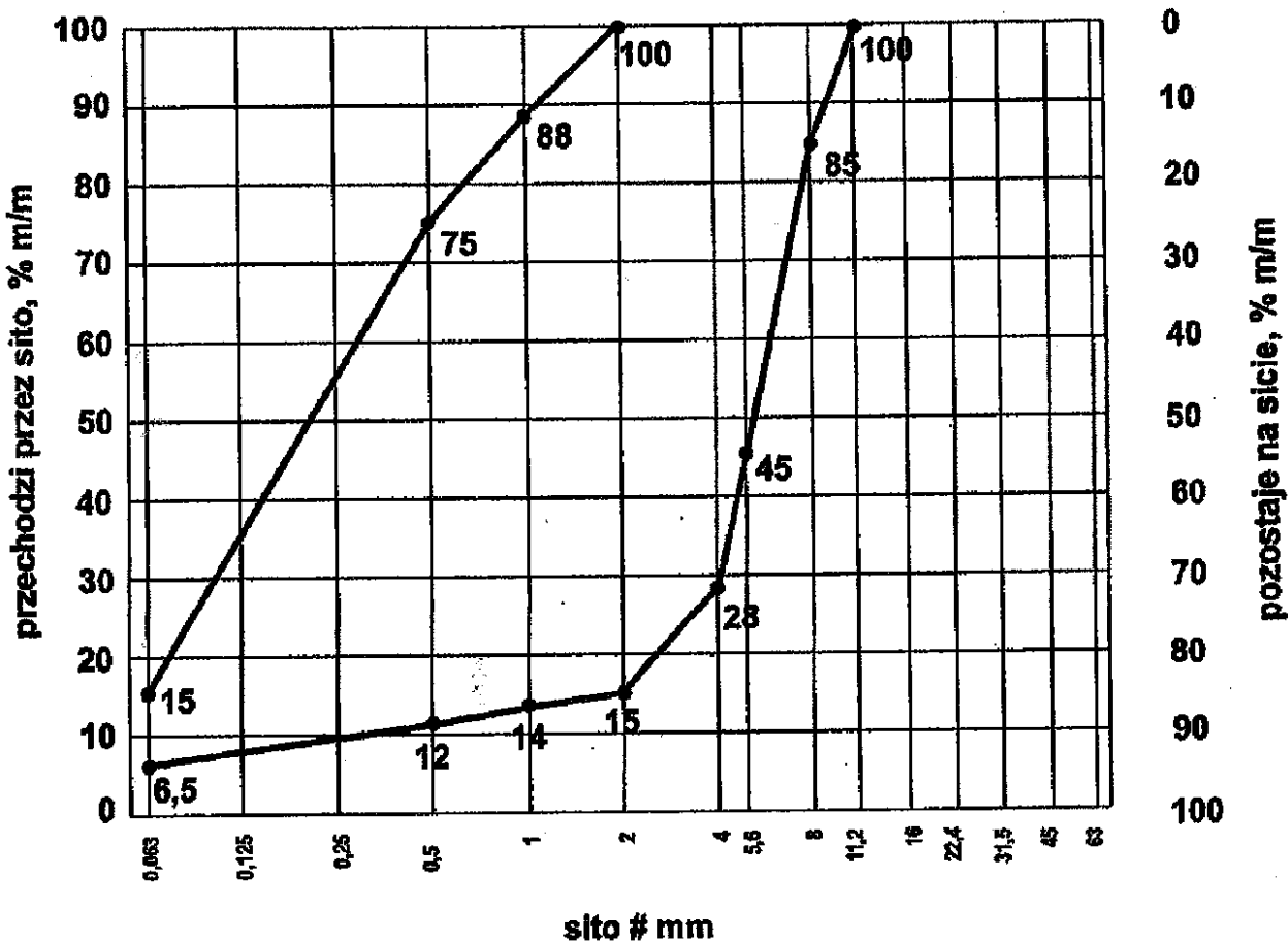
Rys.5. Krzywe graniczne uziarnienia mieszanki mineralnej 0/8 mm
