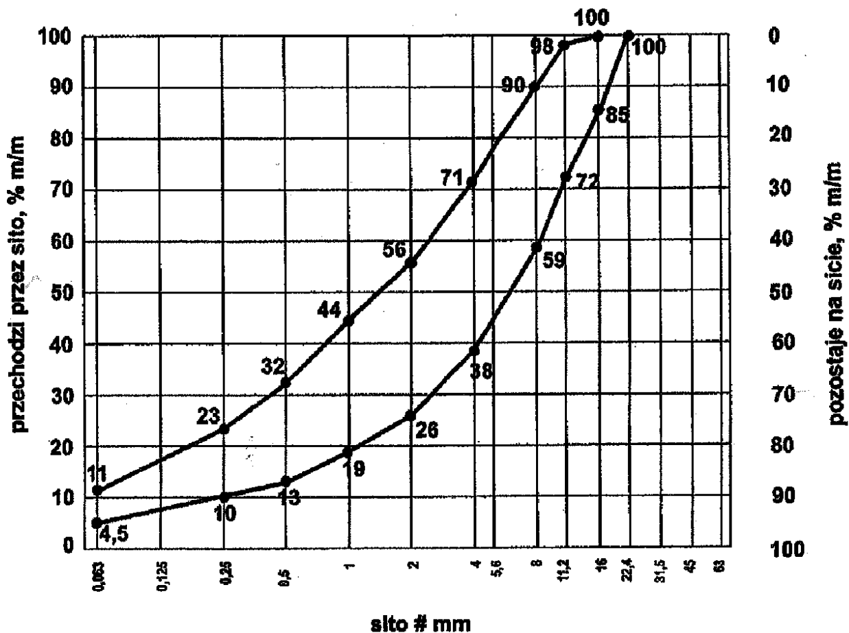
Rys. 3. Krzywe graniczne uziarnienia mieszanki mineralnej 0/16 mm
