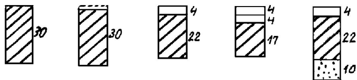
Rys. 4. Przykładowe wybrane konstrukcje nawierzchni utwardzonego pobocza z kruszywą łamaną niezwiązaną
