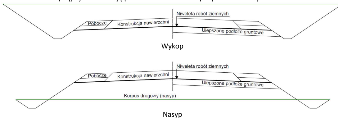
Rysunek 1.1. Lokalizacja niwelety robót ziemnych
